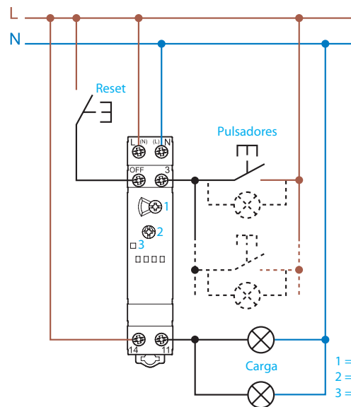
Tipo 14.11 - Cableado de alimentación y carga con la misma fase
