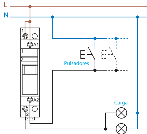
Conexión del mando con alimentación coincidente con la red
