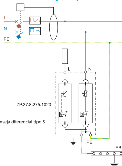
TN-S monofásica aguas abajo del diferencial
