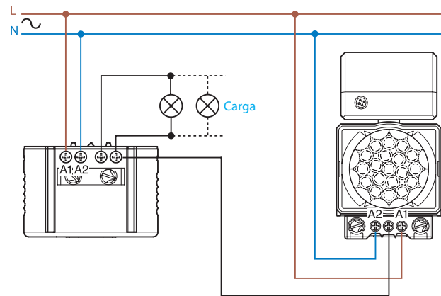
Conexión en paralelo Tipo 18.01/11 con Tipo 18.21/31
