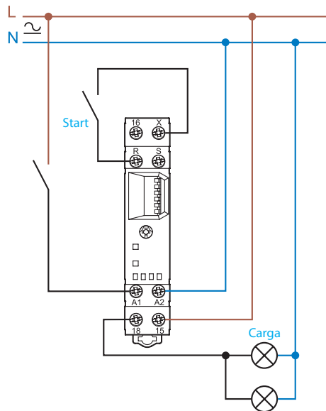
81.01 - Conexión con Start coincidente con la alimentación
