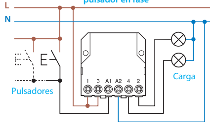
Conexión con señal de mando mediante pulsador en fase
