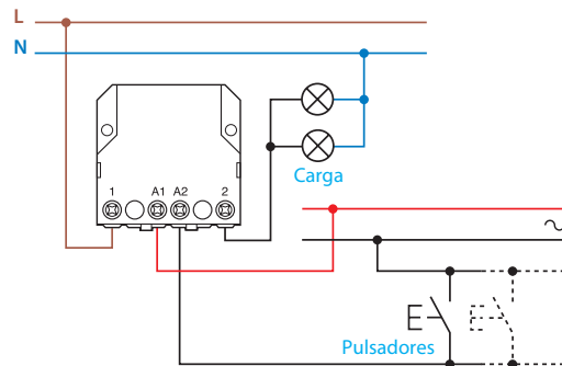
Conexión con mando a muy baja tensión alterna
