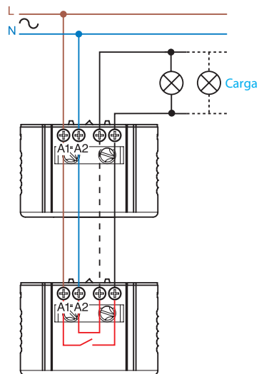
Conexión en paralelo Tipo 18.21/31
