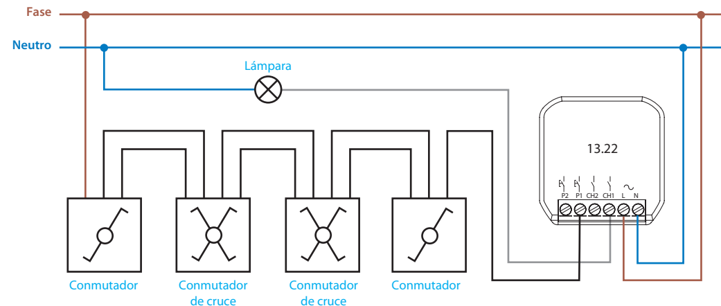
YESLY - función de interruptor Rla (accionado por interruptores)
