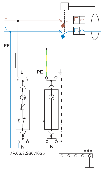
TT monofásica aguas arriba del diferencial
