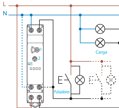
14.01 - Conexión a 4 hilos (pulsador actuando sobre la fase)
