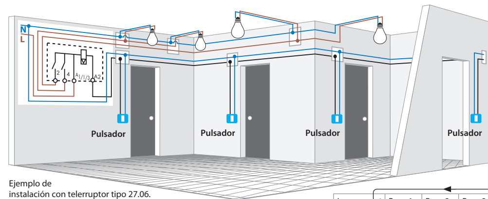
Función ...6, conmutador 3 secuencias — Instalación con telerruptor tipos 20.26 - 26.06 - 27.06 - 27.26
