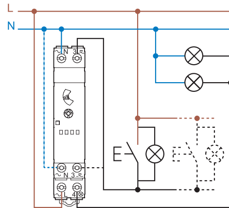
Conexión a 4 hilos
