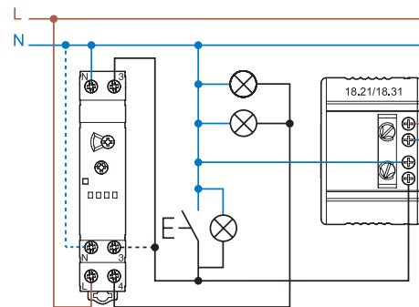
Conexión a 3 hilos (pulsador actuando sobre el neutro) (solo con 18.21.8.230.0300 o 18.31.8.230.0300)
