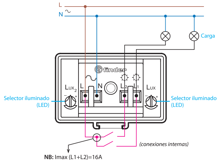
Tipo 10.42 Dos umbrales, dos salidas NA Corte unipolar (F) - 2 NA, 16 A 230 V AC - Alimentación: AC - Montaje en poste o pared
