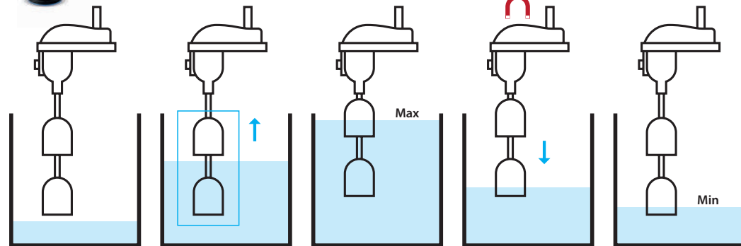
Funciones vaciado/llenado
