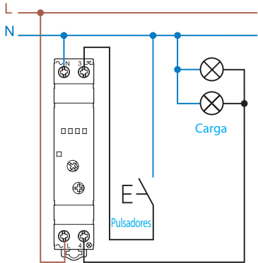
Conexión a 3 hilos (pulsador actuando sobre el neutro)
