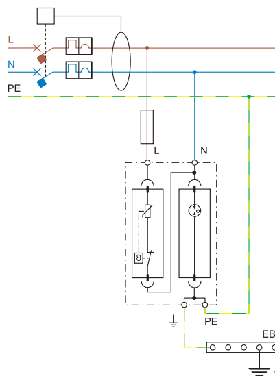
TT o TN-S monofase aguas abajo del diferencial
