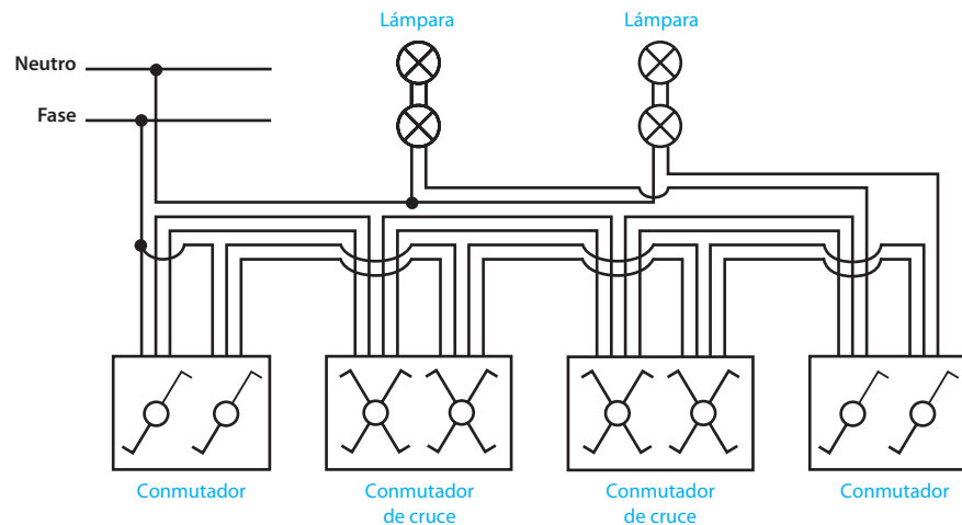
Función ...6, conmutador 3 secuencias — Esquema de conexión instalación tradicional
