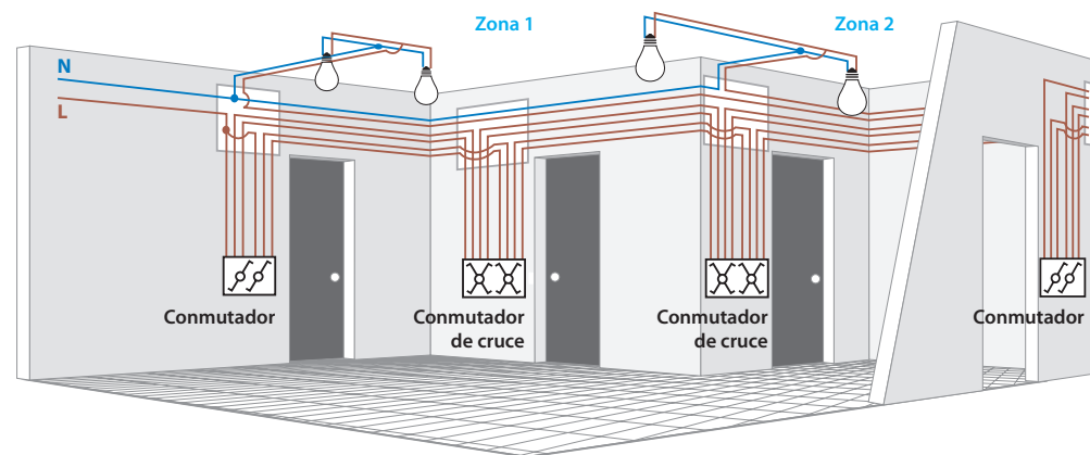
Función ...6, conmutador 3 secuencias — Instalación tradicional
