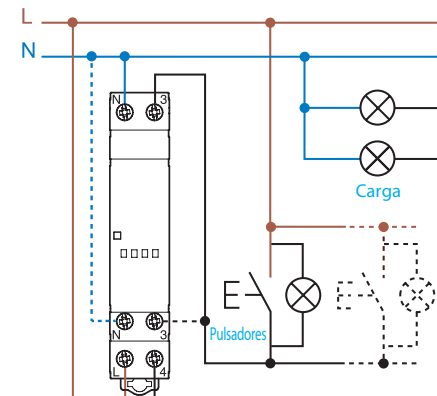
Conexión a 4 hilos (pulsador actuando sobre la fase)
