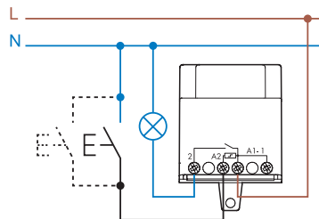
Versión con 1 salida NA
