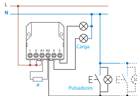
Conexión del mando con alimentación con la red y utilización de pulsadores luminosos
