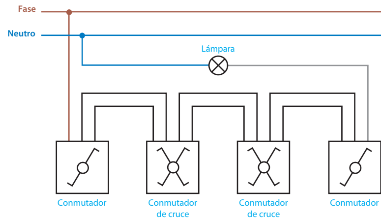
Función ...1, interruptor unipolar — Esquema de conexión instalación tradicional
