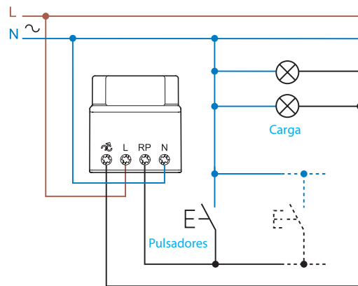
Conexión a 3 hilos (pulsador actuando sobre el neutro)
