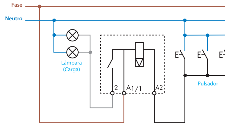
Ejemplo de instalación con telerruptor tipo 27.01.
