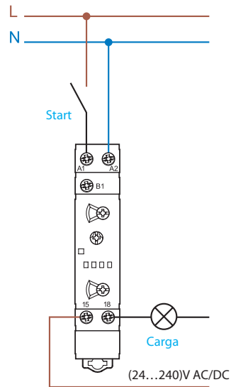
Conexión con mando coincidente con la alimentación (A1)
