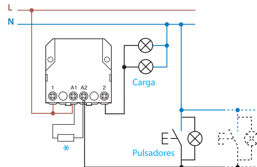
Conexión del mando con alimentación con la red y utilización de pulsadores luminosos
