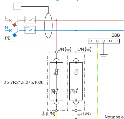
TN-S monofásica aguas abajo del diferencial
