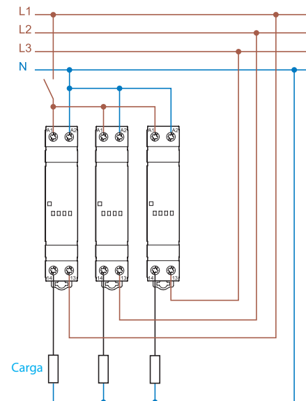
Ejemplo de conexión trifásica (con 3 x 77.01.8.230.8051)
