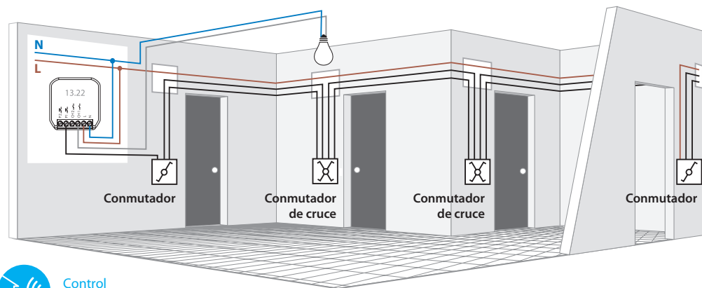
YESLY - Función de conmutador Rla (accionado por interruptores)
