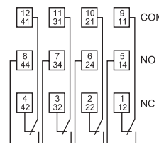
4 contactos conmutados
