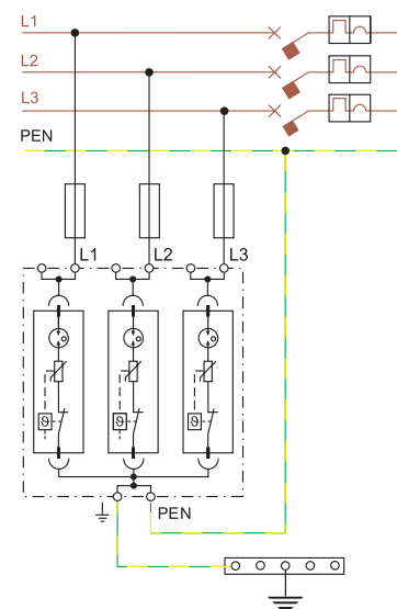
TN-C trifásica aguas arriba del diferencial
