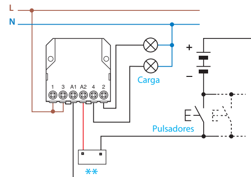
Conexión con mando en corriente continua
