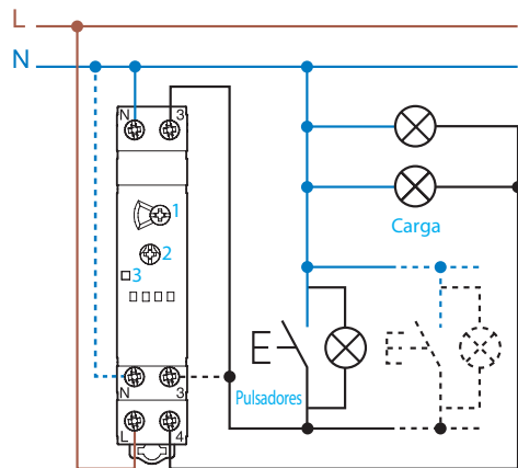
14.01 - Conexión a 3 hilos (pulsador actuando sobre el neutro)
