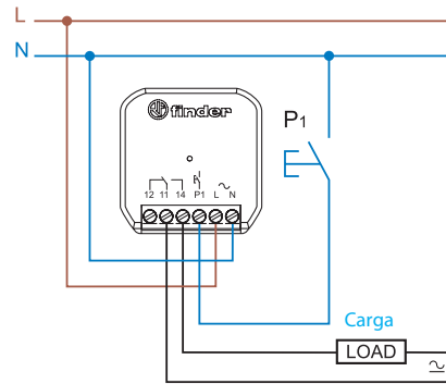
Cableado con pulsador a neutro
