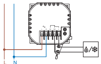
Esquema de conexión estándar
