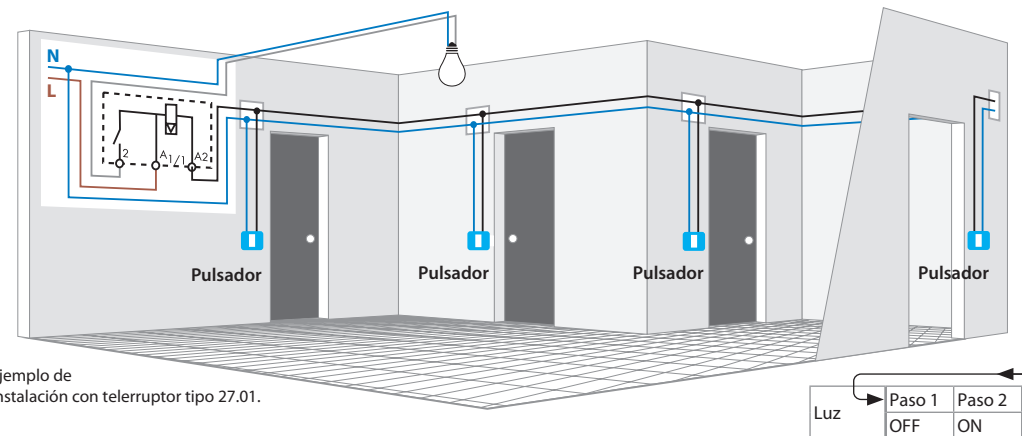
Función ...1, interruptor unipolar — Instalación con telerruptor tipos 20.21 - 26.01 - 27.01 - 27.21 - 13.81 - 13.91
