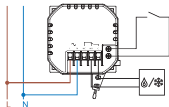
Contacto seco externo para modo nocturno
