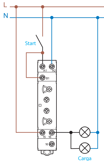
Conexión con mando coincidente con la alimentación (A1)
