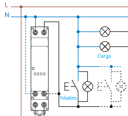
Conexión a 3 hilos (pulsador actuando sobre el neutro)
