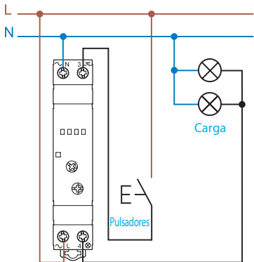
Conexión a 4 hilos (pulsador actuando sobre la fase)
