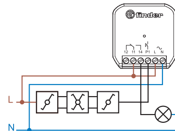
Instalación smart
