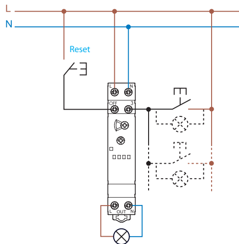
13.62.8.230.0001 Conexión a 4 hilos
