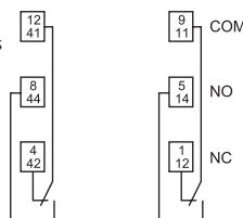
2 contactos conmutados
