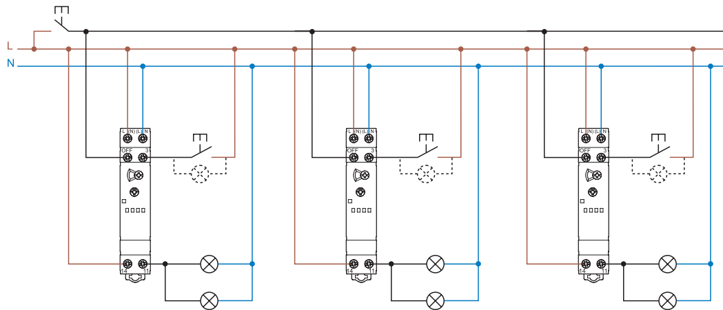
Ejemplo de conexionado con más 13.61.8.230.0000 con pulsador de apagado centralizado Conexión a 4 hilos (pulsador actuando sobre la fase)
