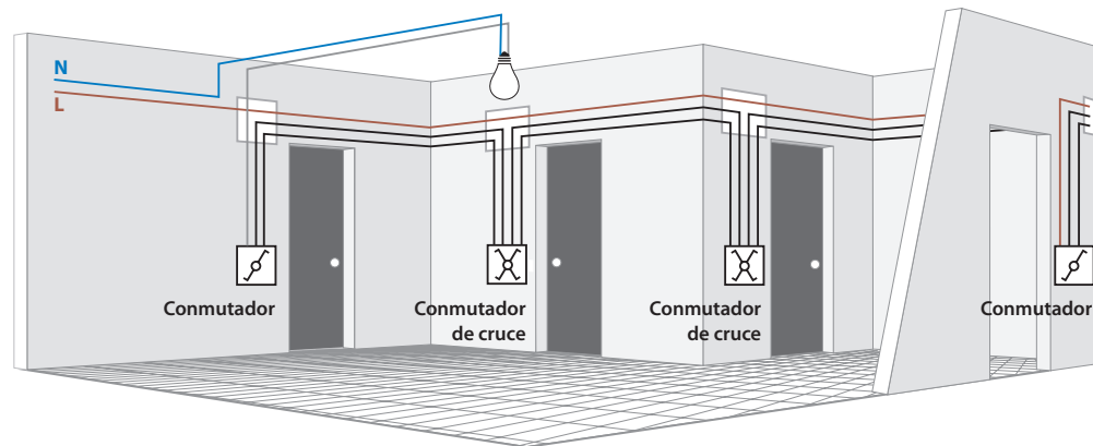
Función ...1, interruptor unipolar — Instalación tradicional
