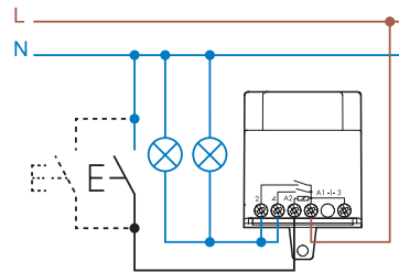
Versión con 2 salidas NA
