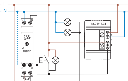
Conexión a 4 hilos (pulsador actuando sobre la fase) (solo con 18.21.8.230.0300 o 18.31.8.230.0300)
