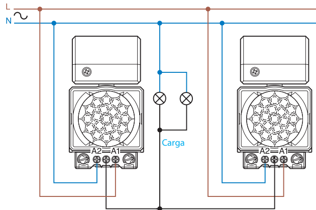
Conexión en paralelo Tipo 18.01/11
