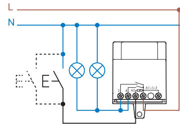
Versión con 2 salidas NA
