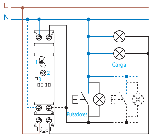
14.71 - Conexión a 3 hilos (pulsador actuando sobre el neutro)
