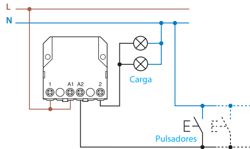
Conexión del mando con alimentación coincidente con la red
