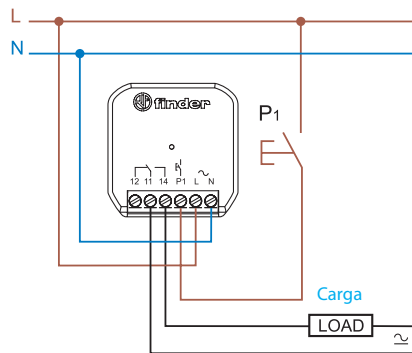
Cableado con pulsador a fase
