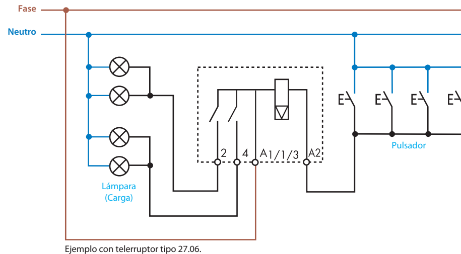
Función ...6, conmutador 3 secuencias — Esquema de conexión con telerruptor
