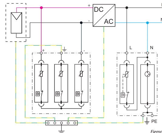
Ejemplo de instalación
