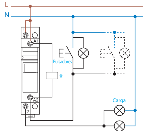
Conexión del mando con alimentación coincidente con la red y utilización de pulsadores luminosos
