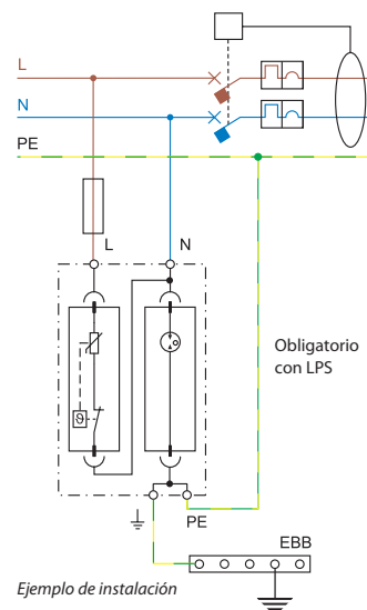
TT monofase aguas arribadel diferencial
