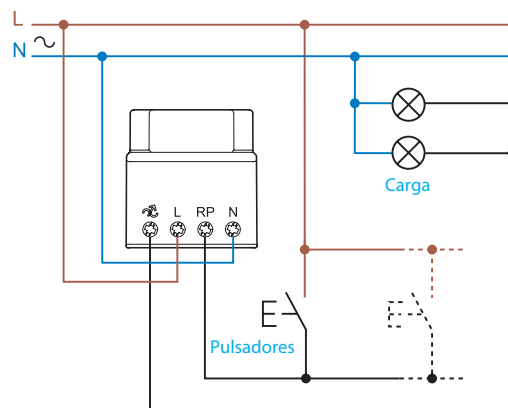
Conexión a 4 hilos (pulsador actuando sobre la fase)
