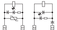
AC DC +
