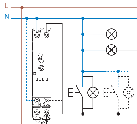
Conexión a 3 hilos
