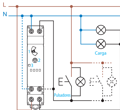
14.71 - Conexión a 4 hilos (pulsador actuando sobre la fase)
