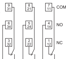
3 contactos conmutados
