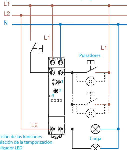
Tipo 14.11 - Cableado de alimentación y carga con distinta fase
