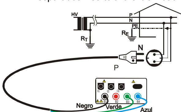
Conexión instrumento para Medida de la impedancia del bucle de avería en un sistema Monofásico o Bifásico 230V
