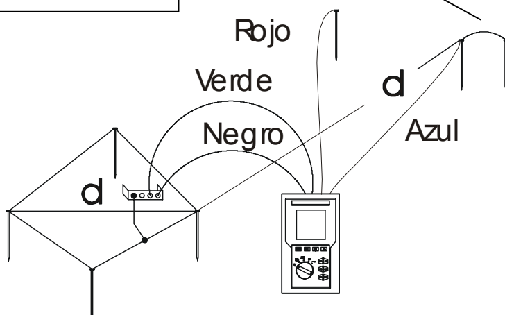
Fig.: medida de la resistencia de tierra con método voltiamperimétrico para conexiones con tierra de pequeñas dimensiones
