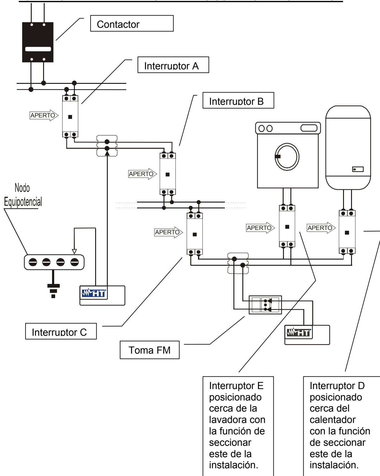
Medidas de aislamiento sobre una instalación.
