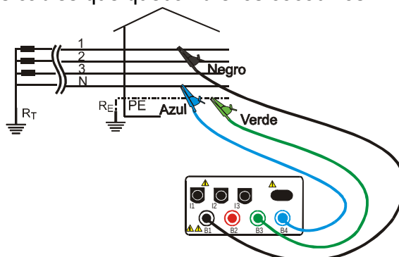
Conexión instrumento para Medida de la impedancia del bucle de avería en un sistema Trifásico 400V con neutro
