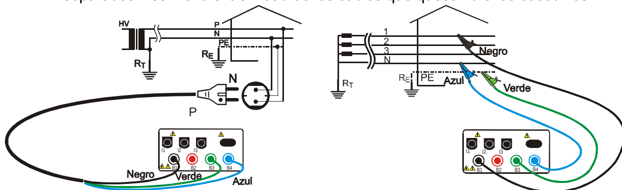
Conexión instrumento para Medida de la impedancia del bucle de avería en un sistema Trifásico 400V con neutro
