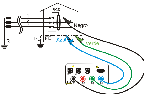
Conexión instrumento para Verificación Diferencial Trifásica 400V + PE (no N)
