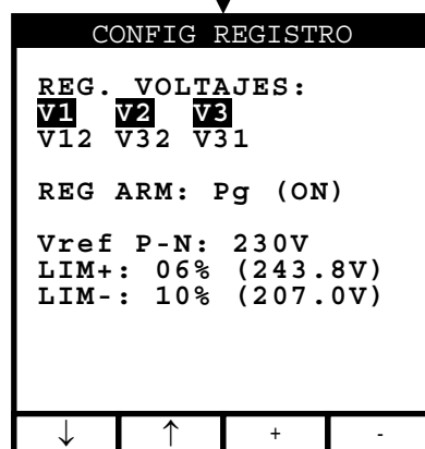
Ejemplo de pantalla de la 2ª Pagina del "MENU" en modalidad Trifásico 4 hilos con mensaje "REG ANOM" seleccionado
